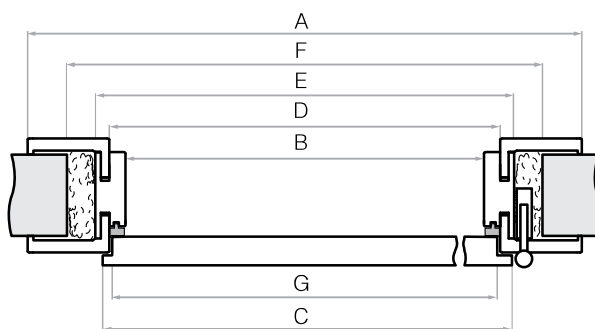
NÁKRES ZÁRUBNE
