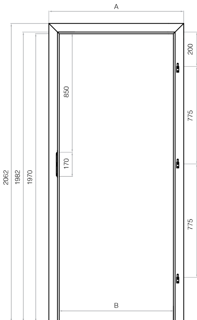
ČELNÝ NÁHĽAD
