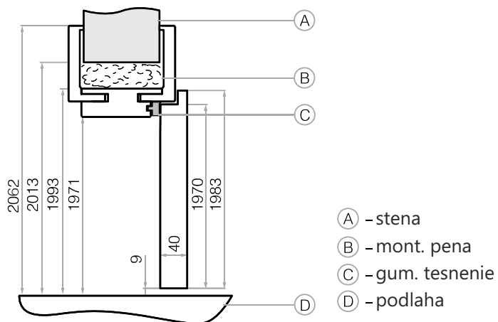
NÁKRES OBLOŽKOVEJ ZÁRUBNE
